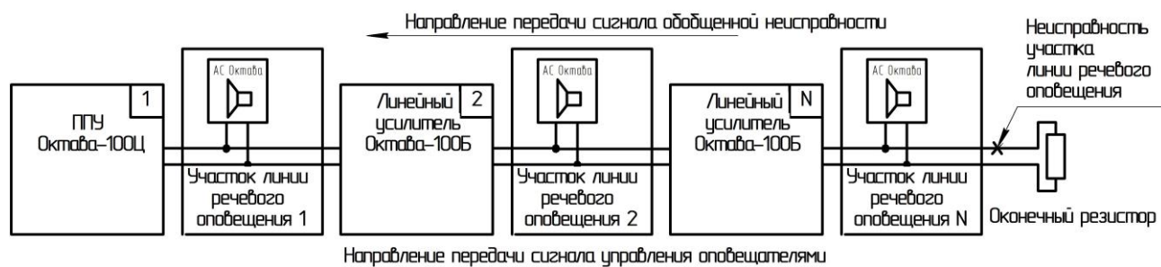
Рисунок 3.2 - Схема передачи сигнала «Неисправность» по линии речевого оповещения
