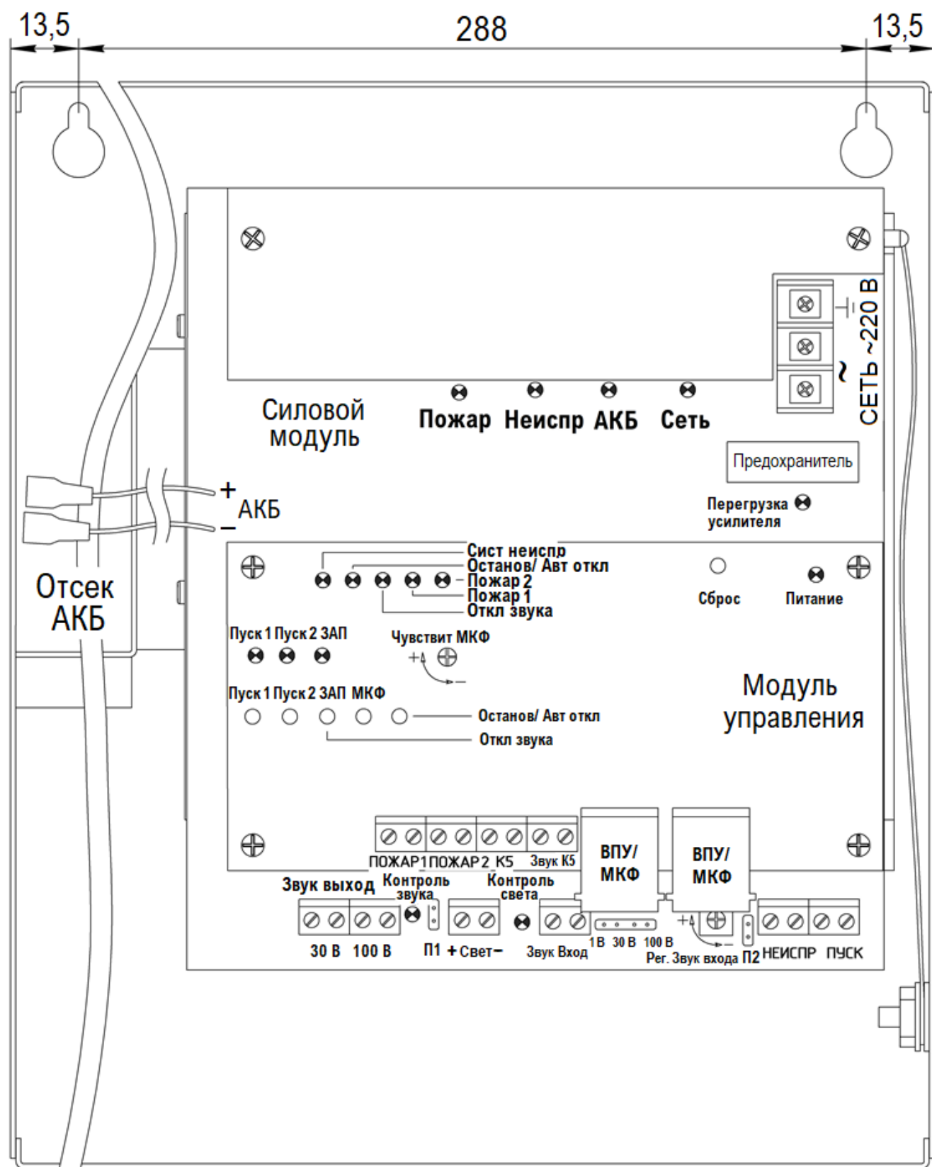
Рисунок 2.1 - Общий вид ППУ со снятой крышкой
